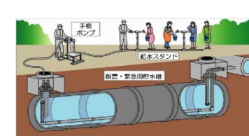
緊急貯水槽
